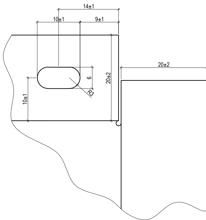
Узел Д - Угол кассеты
